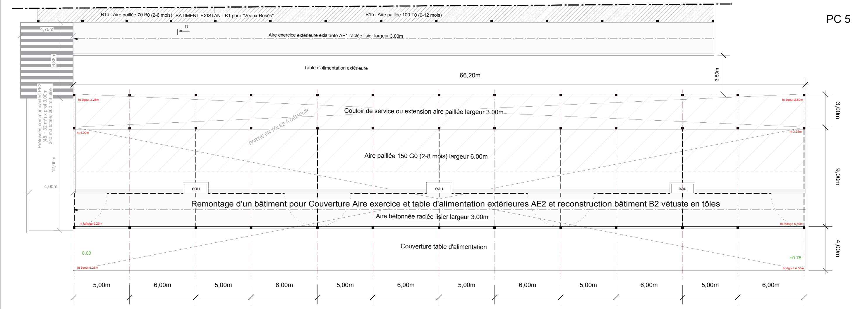
VUE EN PLAN RECONSTRUCTION BÂTIMENT B2 PC 5
