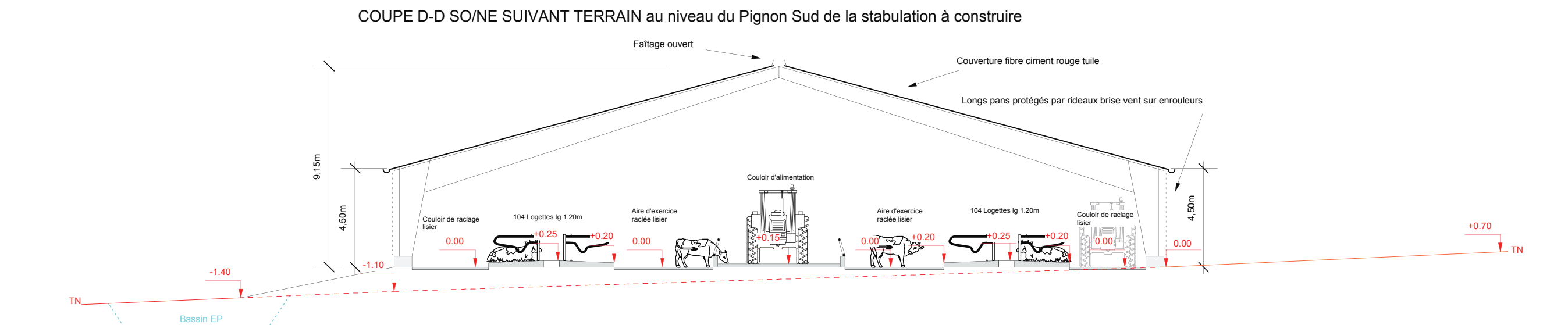
COUPE D-D S'ONNE SUIVANT TERRAIN au niveau du Pignon Sud de la stabulation à construire
